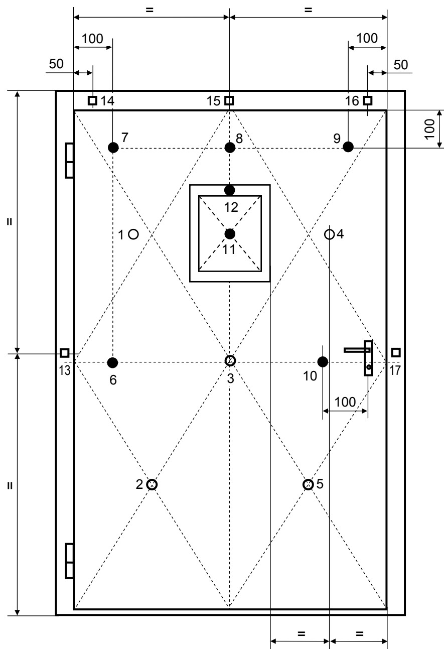
Рисунок 21 — Схема установки термодатчиков на неотапливаемой поверхности распашной одностворчатой двери с частичным остеклением
