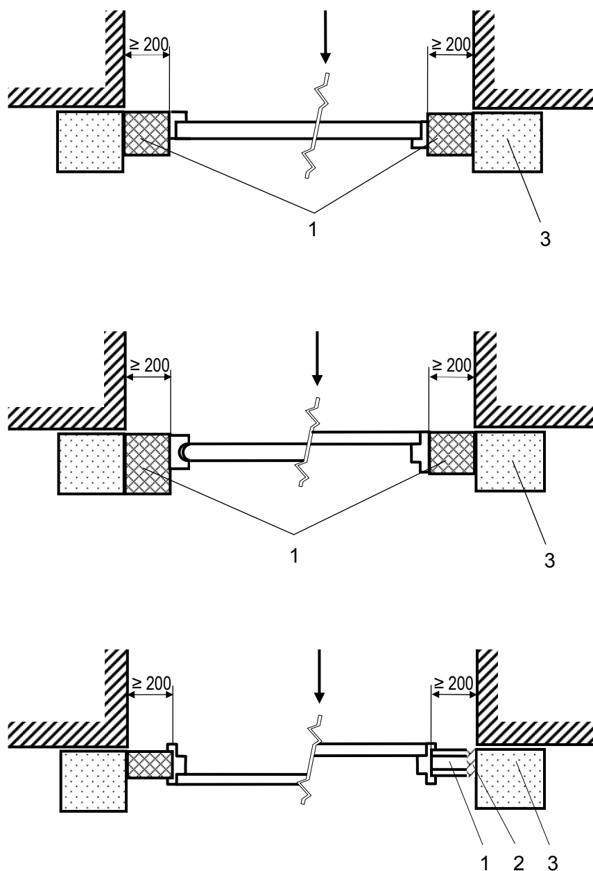
1 — фрагмент ограждающей конструкции; 2 — теплоизоляционная прокладка; 3 — рама для установки фрагмента ограждающей конструкции; ↓ — направление теплового воздействия
